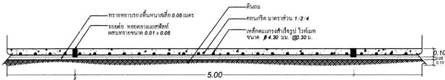
แบบขยายรูปตัด A - A
