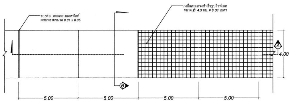
แบบแปลน ขนาดจริง 1:100
